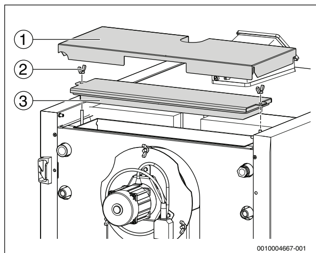
Obr. 30 Čisticí otvor spalínového kanálu
