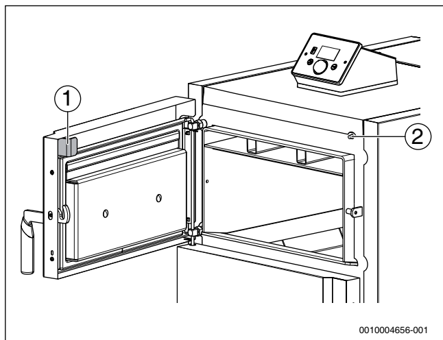
Obr. 18 Dveřní spínač
