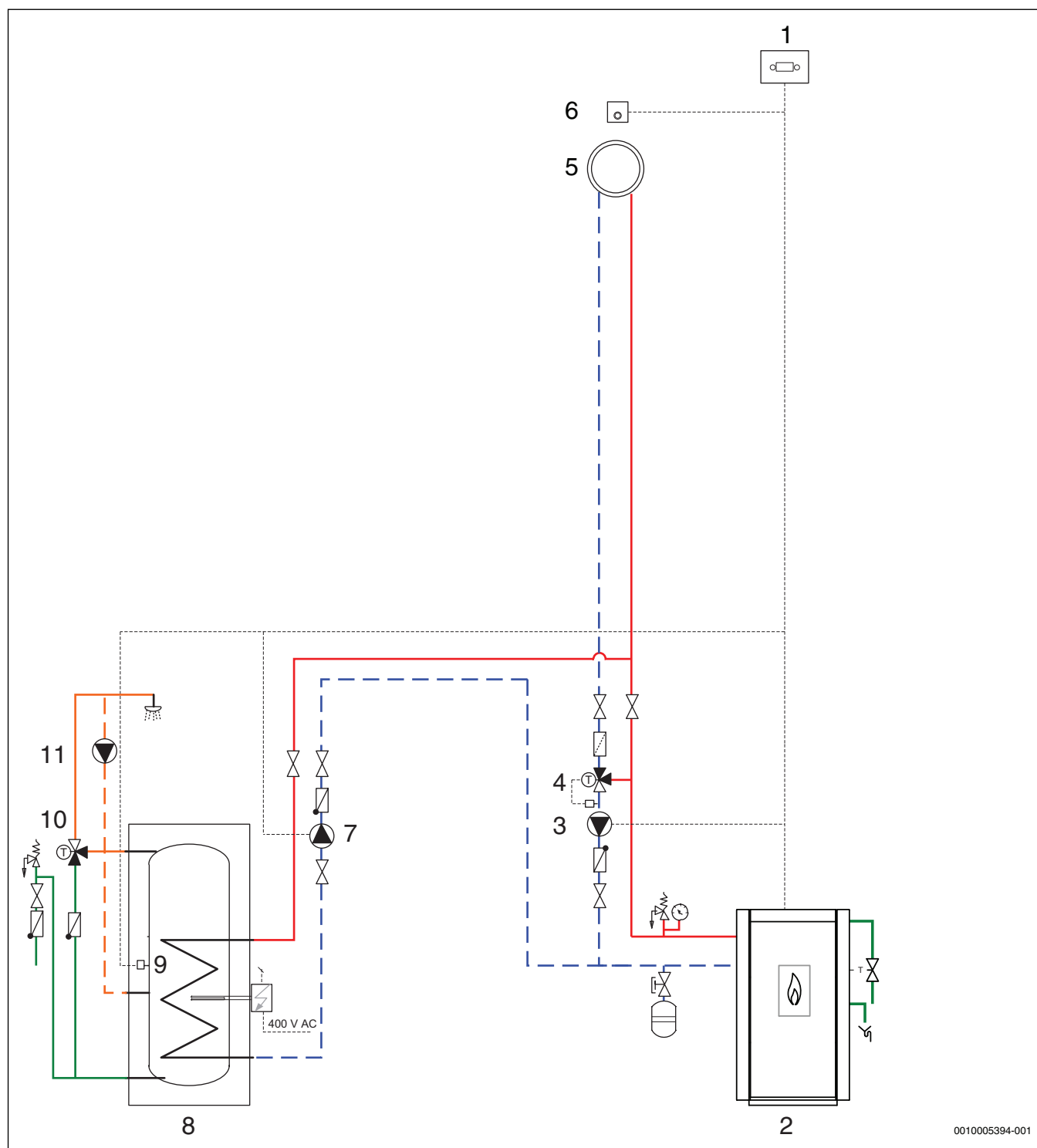
Obr. 46 Příklad zařízení 2 se zvýšením teploty vratné vody, cirkulačním čerpadlem TUV, zásobníkem teplé vody a nesměšovaným otopným okruhem
