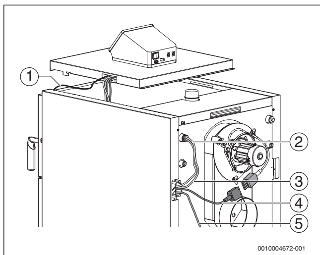
Obr. 21 Protažení kabelů a kabelů čidel krytem kotle
