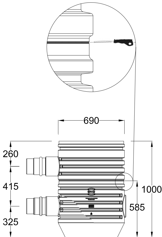
VS-Verteilermodul DN 600 330361
