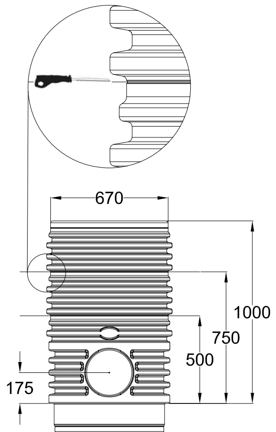
VS-Zwischenstück 1000 DN 600 371015/ 371016
