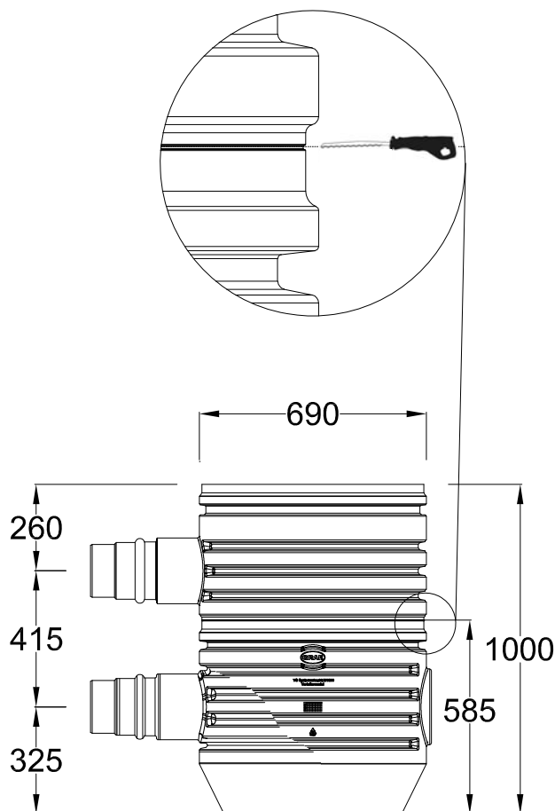
Regard de répartition DN 600 330361
