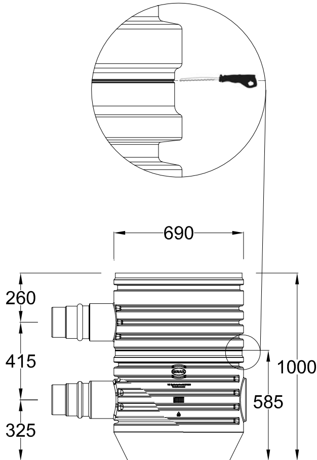
Módulo de distribución de la arqueta modular 330361
