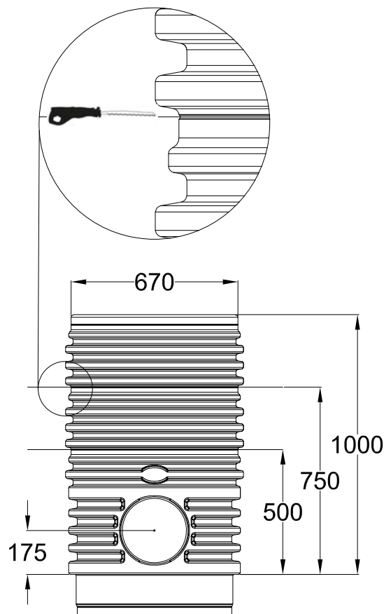
Rallonge por regard 1000 DN 600 371015/ 371016
