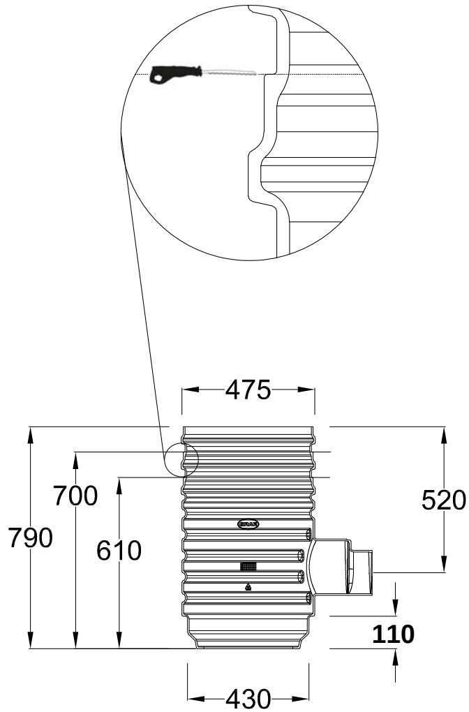
Infiltration inlet module DN 400 330339
