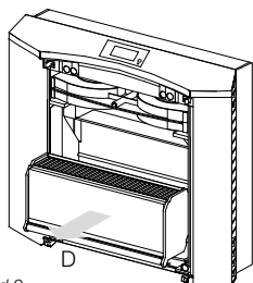
Bild 9 Alten Filter herausnehmen
