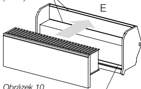
Obrázek 10 Vložení nového filtru hliníková hrana (3)
