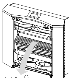
Obrázok 8 C Vyklonenie tepelného výmenníka
