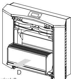
Obrázek 9 Vyjmutí starého filtru ven
