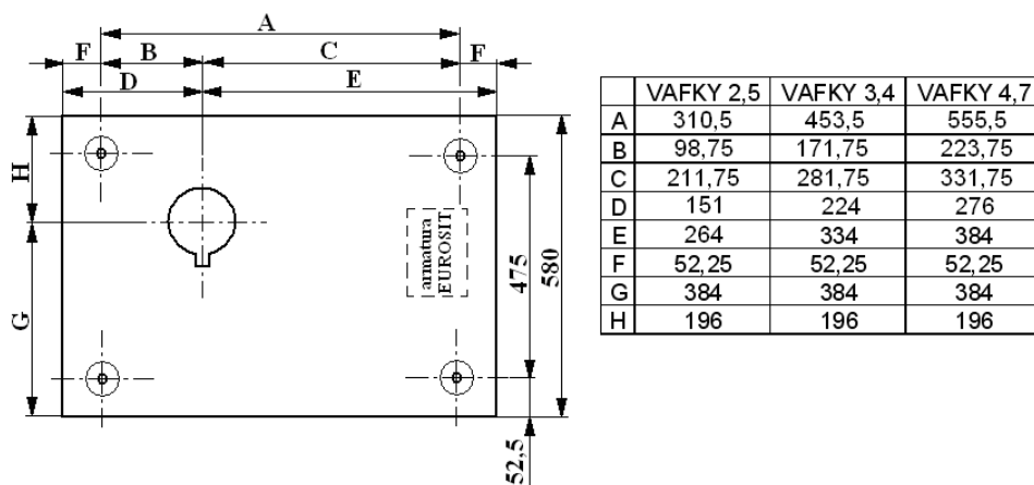
Rozměrový náčrtek - zadní strana topidla
