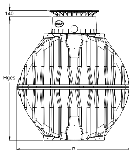
Carat S avec Mini dôme de la cuve
