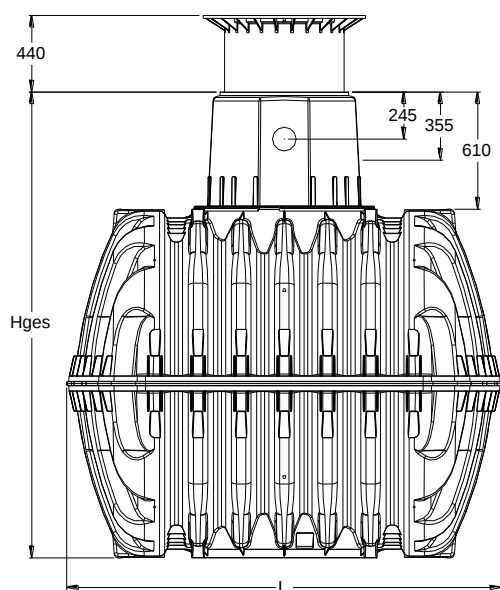
Carat S avec Maxi dôme de la cuve
