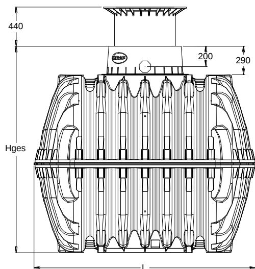
Carat S avec Mini dôme de la cuve
