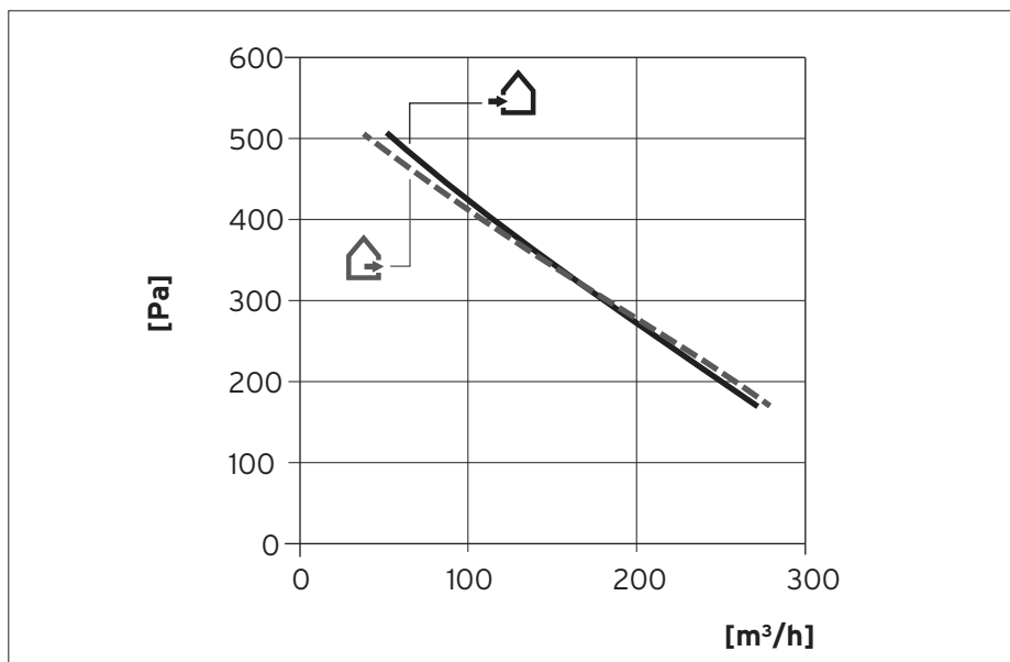
Graf výkonu rekuperační jednotky VAR 260/4
