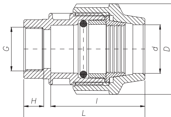
FEMALE ADAPTOR ANSCHLUSSVERSCHRAUBUNG MIT INNENGEWINDE МУФТА С ВНУТРЕННЕЙ РЕЗЬБОЙ
